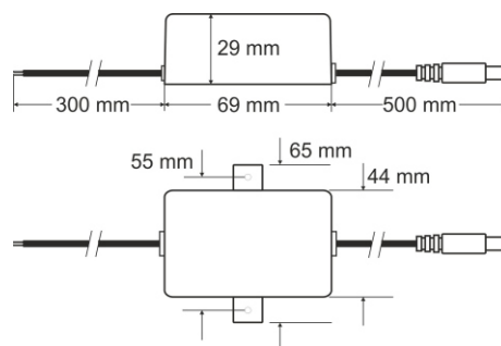
Rys. 1 Widok mechaniczny zasilacza.
