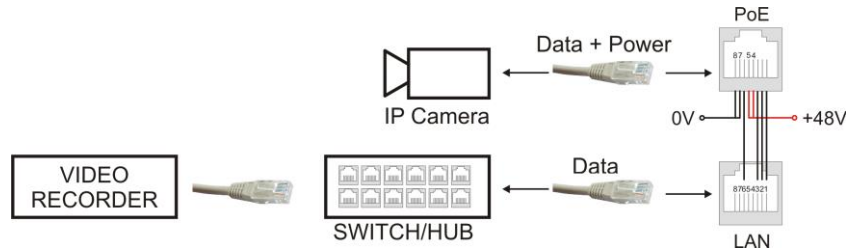
Rys. 4. Schemat podłączenia urządzeń do złącz LAN oraz POE.
