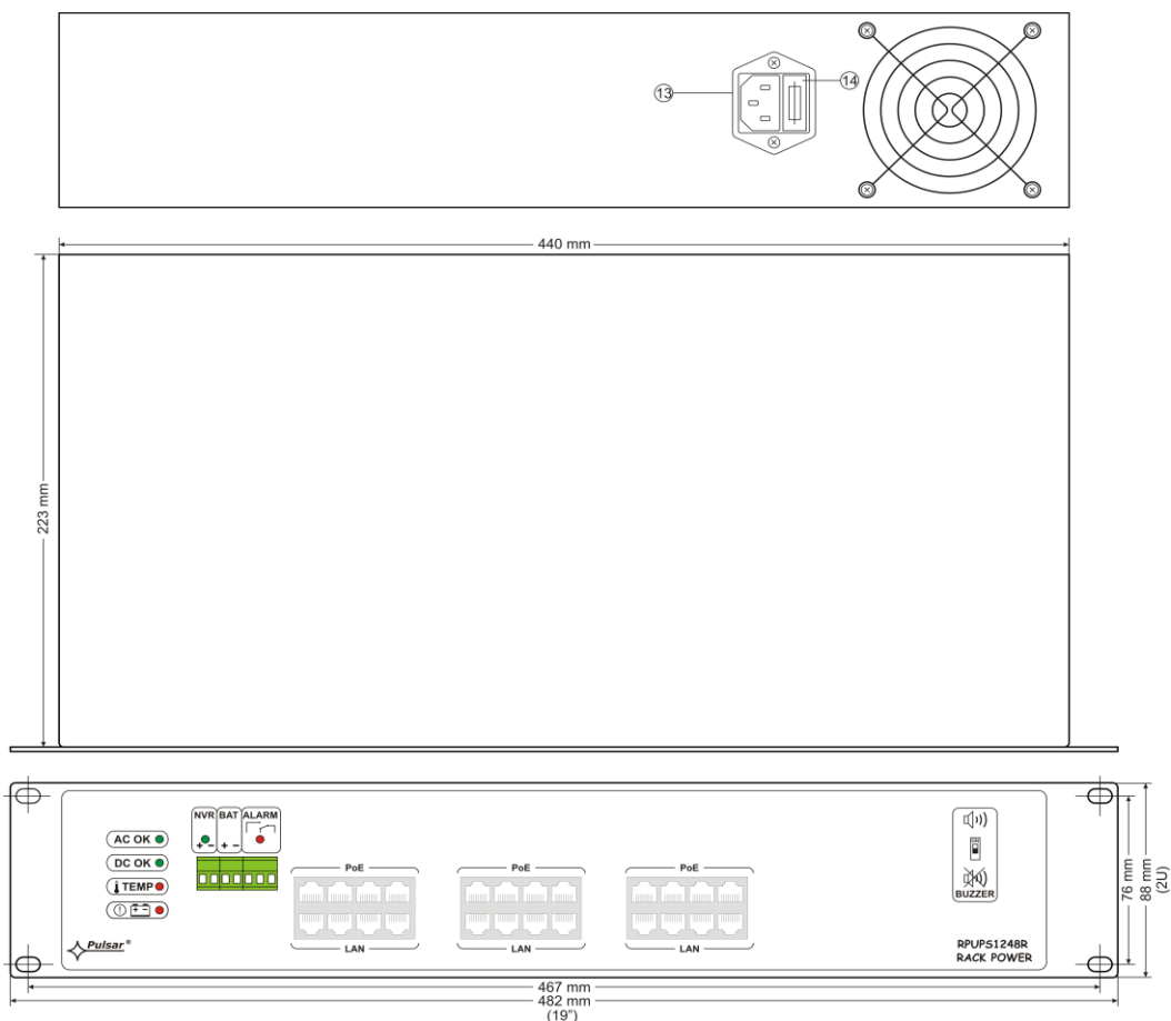
Rys.3. Widok zasilacza.
