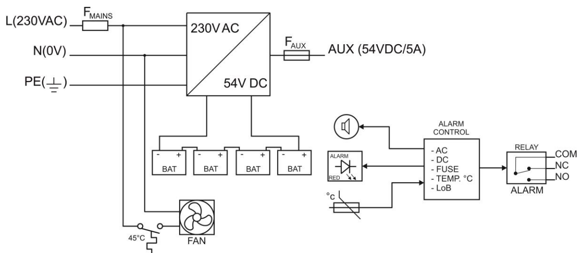
Rys.1. Schemat blokowy zasilacza.
