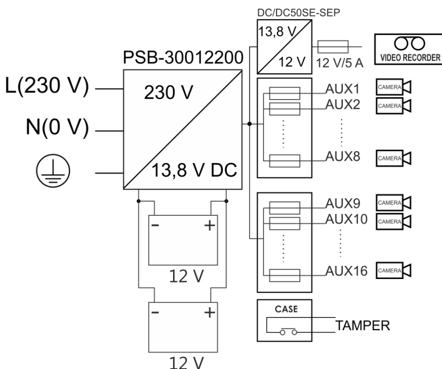
Rys.1. Schemat blokowy zasilacza.
