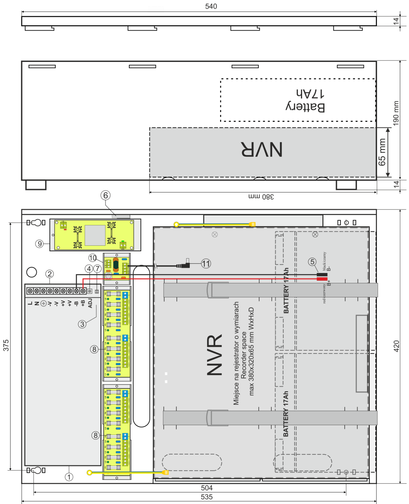
Rys. 4. Widok zasilacza.
