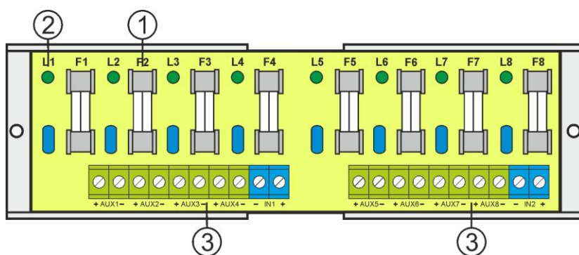
Rys.2. Widok modułu bezpiecznikowego LB8.
