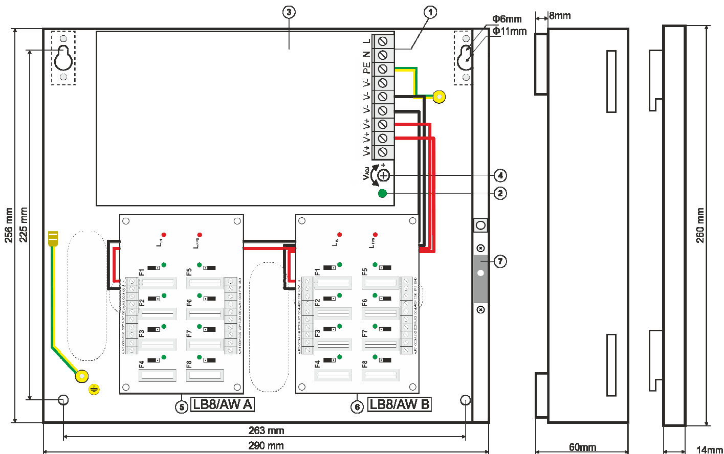
Rys.3. Widok zasilacza.
