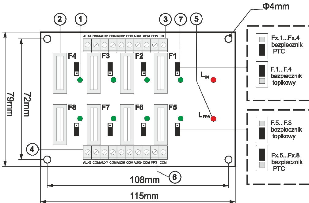
Rys. 2. Widok płyty PCB zasilacza.
