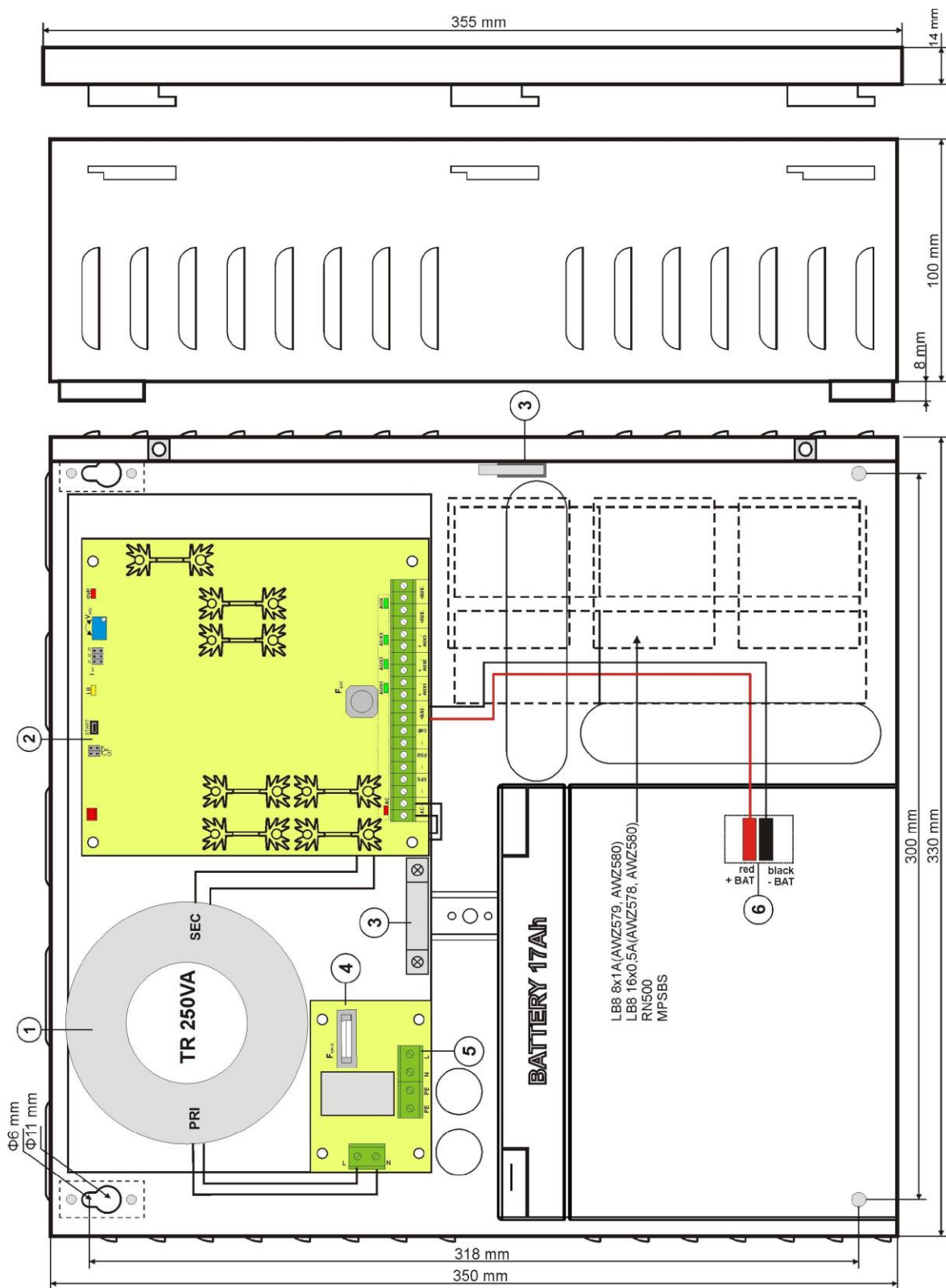
Rys.3. Widok zasilacza.
