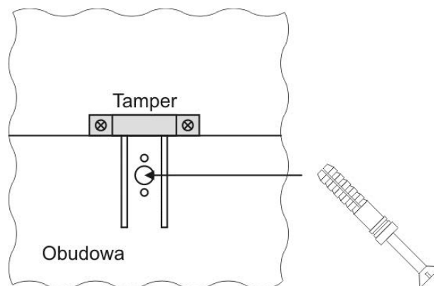
Rys. 4. Montaż uchwyty tampera antysabotażowego.
