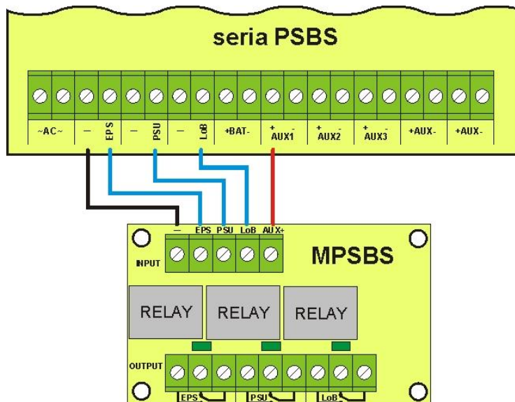
Rys. 6. Schemat podłączenia modułu MPSBS.
