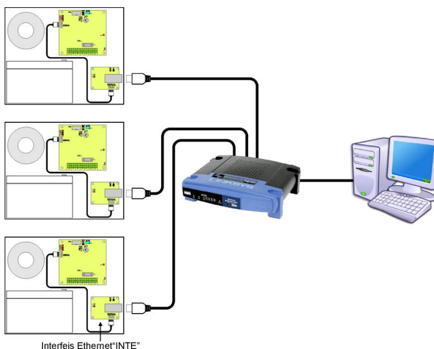
Rys. 25. Komunikacja Ethernet z wykorzystaniem interfejsu Ethernet „INTE”.
