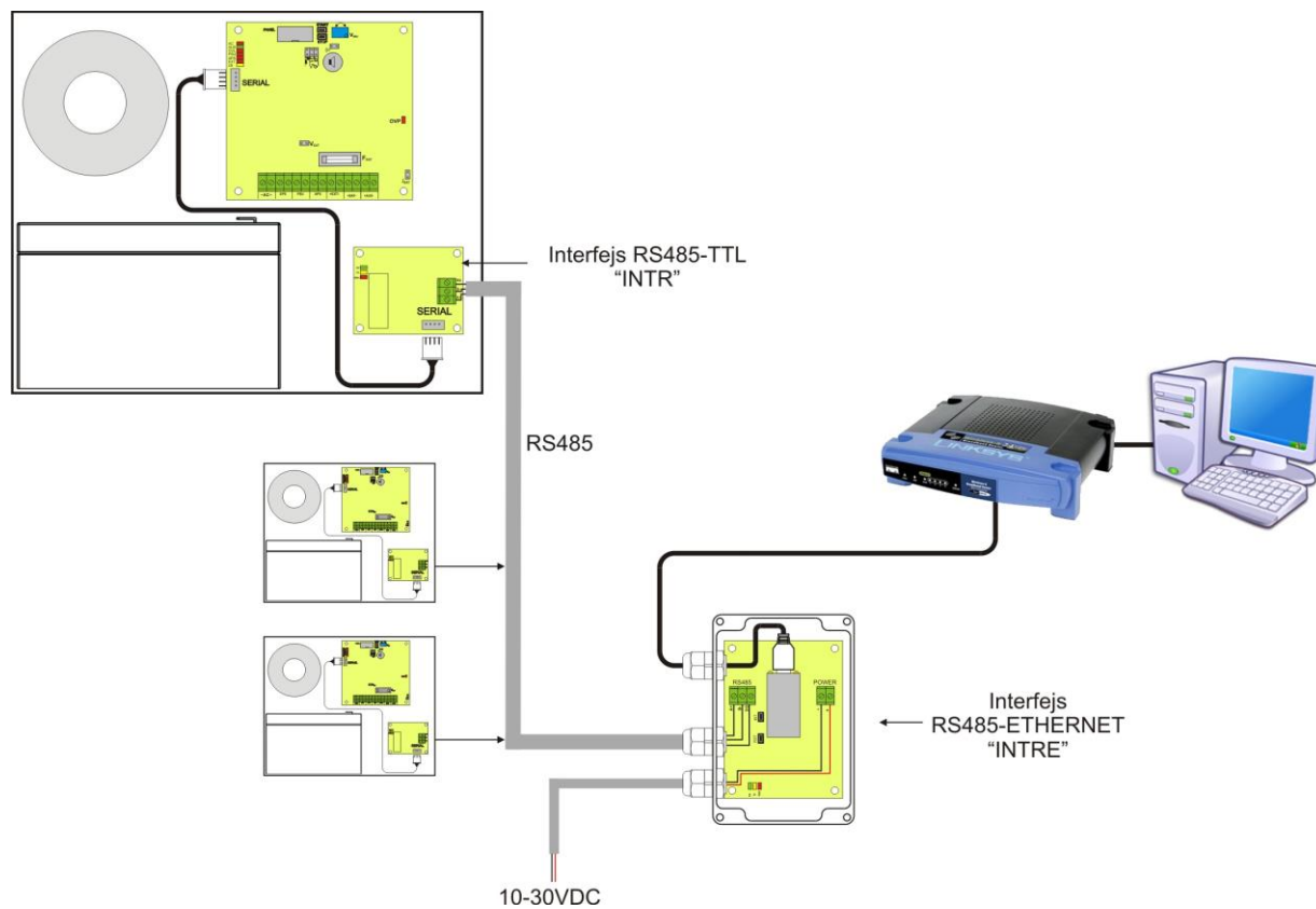
Rys. 26. Komunikacja Ethernet z wykorzystaniem interfejsu RS485-Ethernet „INTRE”.
