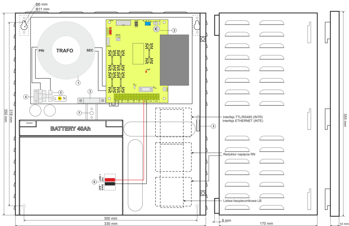
Rys.3. Widok zasilacza.
