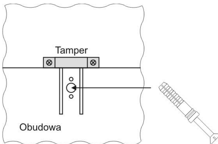
Rys. 4. Montaż uchwyту tampera antysabotażowego.
