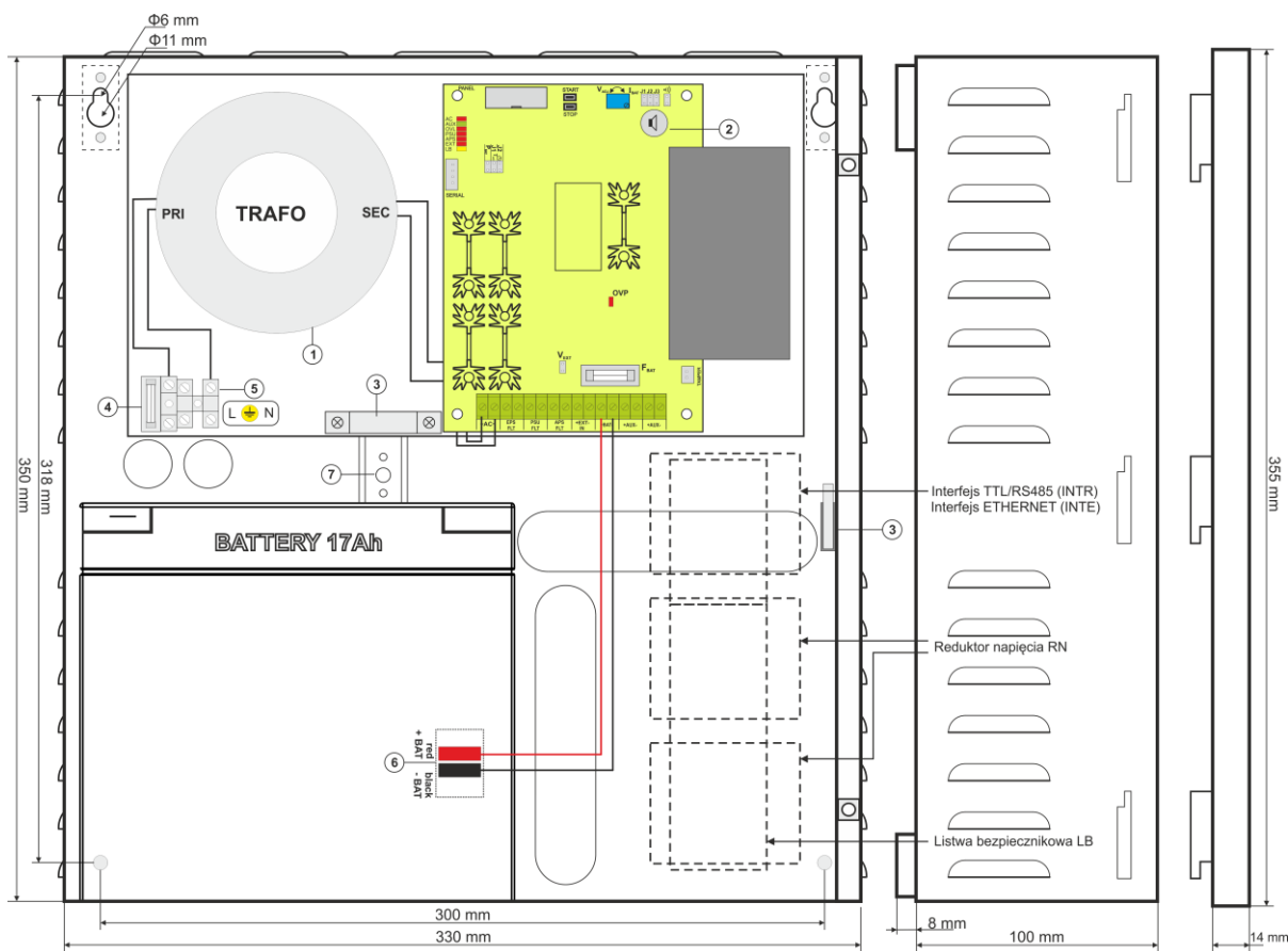
Rys.3. Widok zasilacza.
