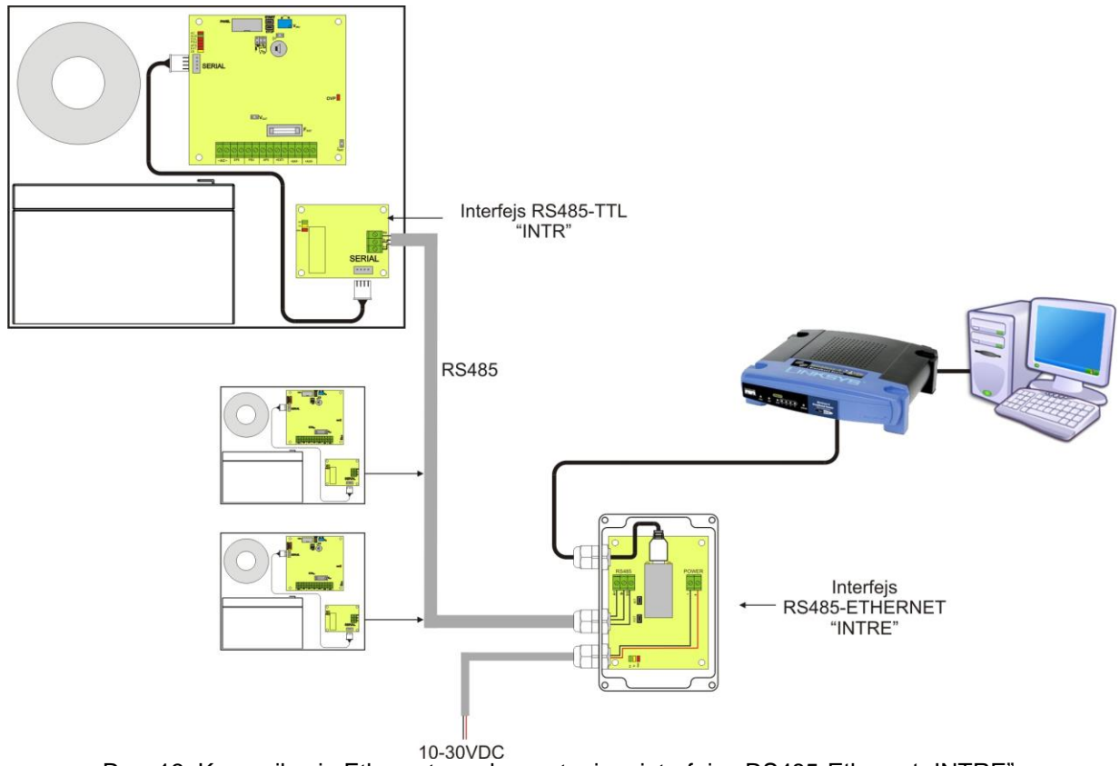
Rys. 13. Komunikacja Ethernet z wykorzystaniem interfejsu RS485-Ethernet „INTRE”.
