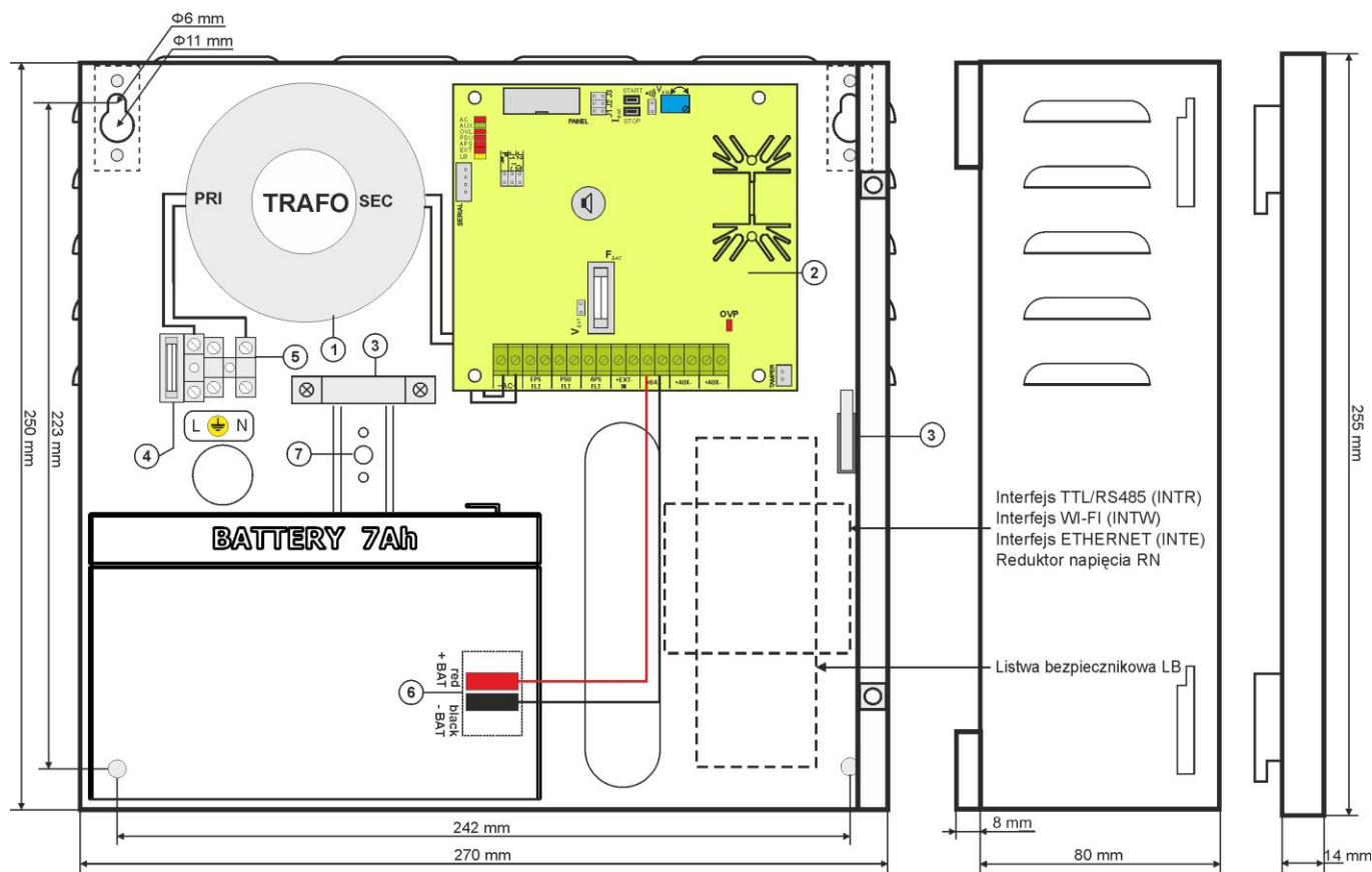
Rys.3. Widok zasilacza.
