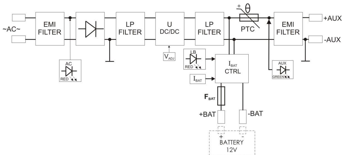
Rys.1. Schemat blokowy modułu zasilacza.
