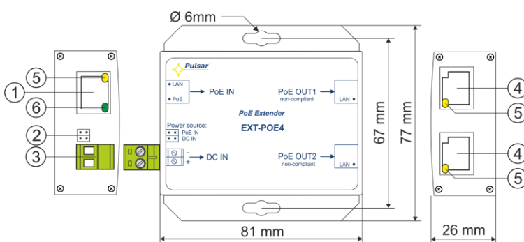
Rys.1. Rysunek urządzenia.
