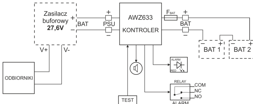
Rys.1. Schemat blokowy kontrolera.
